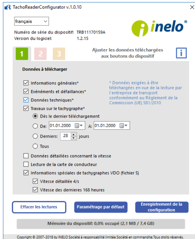
Fig. Fenêtre de configuration de l'appareil: TachoReader Basic.
